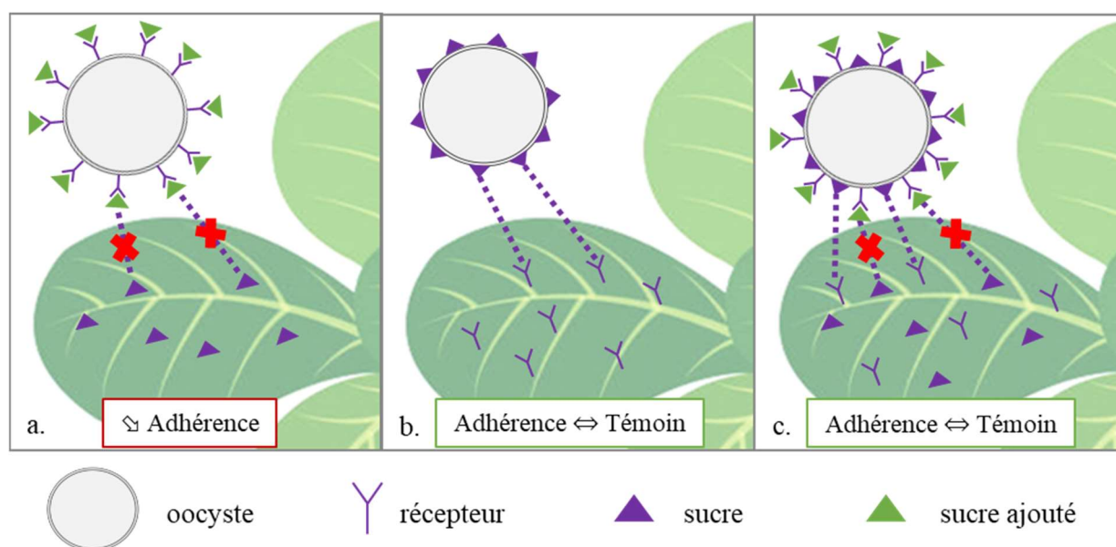
Figure 39 – Schémas des interactions possibles entre le parasite et la mêche après saturation des récepteurs sur l'oocyste par un sucre impliqué dans l'adhérence selon la localisation des récepteurs.
